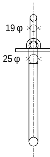
取付け金具詳細図
