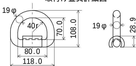
取付け金具詳細図
